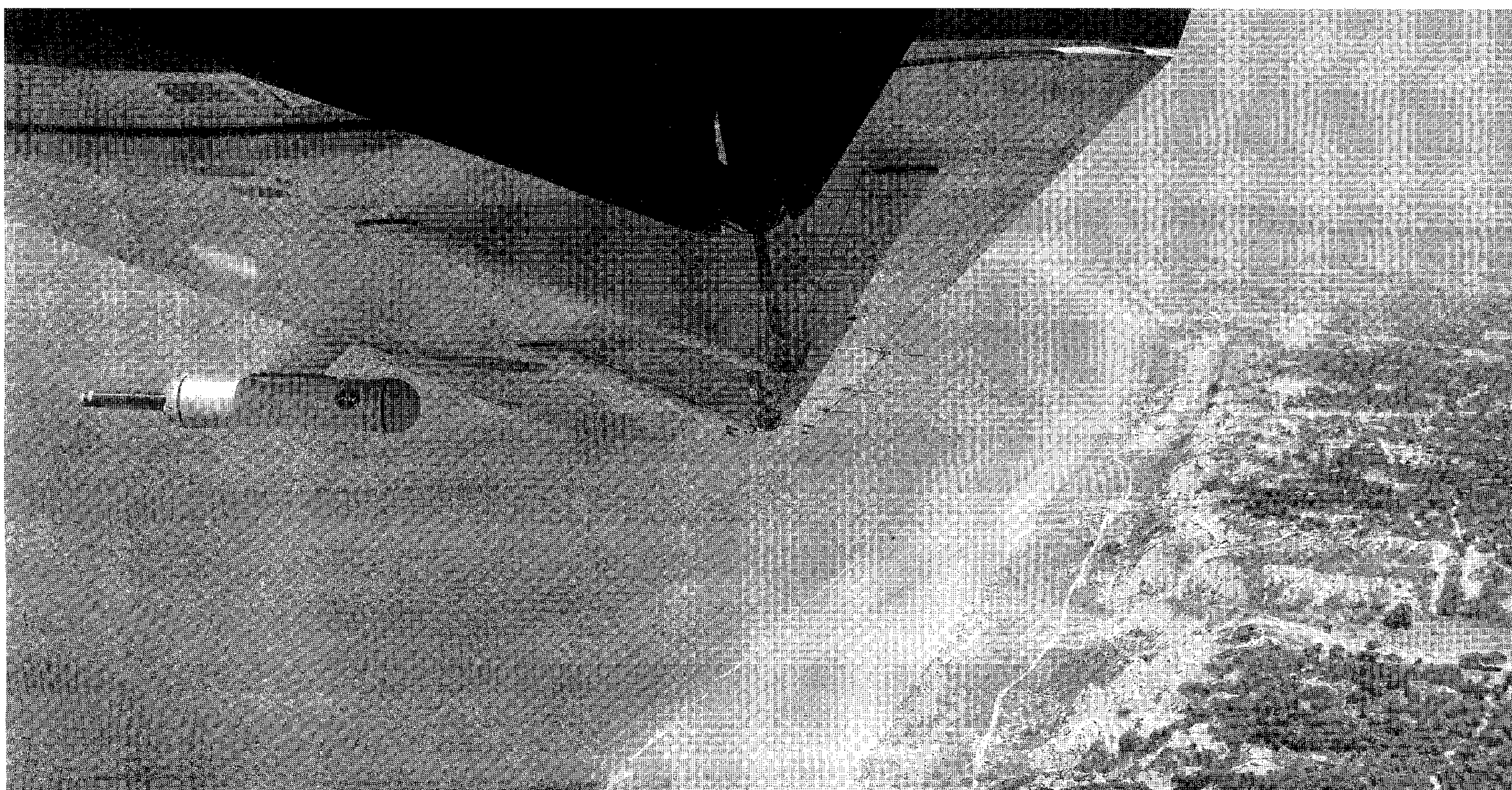
Medidor situado bajo el ala del avión C212 con el que el INTA realiza pruebas atmosféricas de partículas saharianas en la provincia de Huelva.
