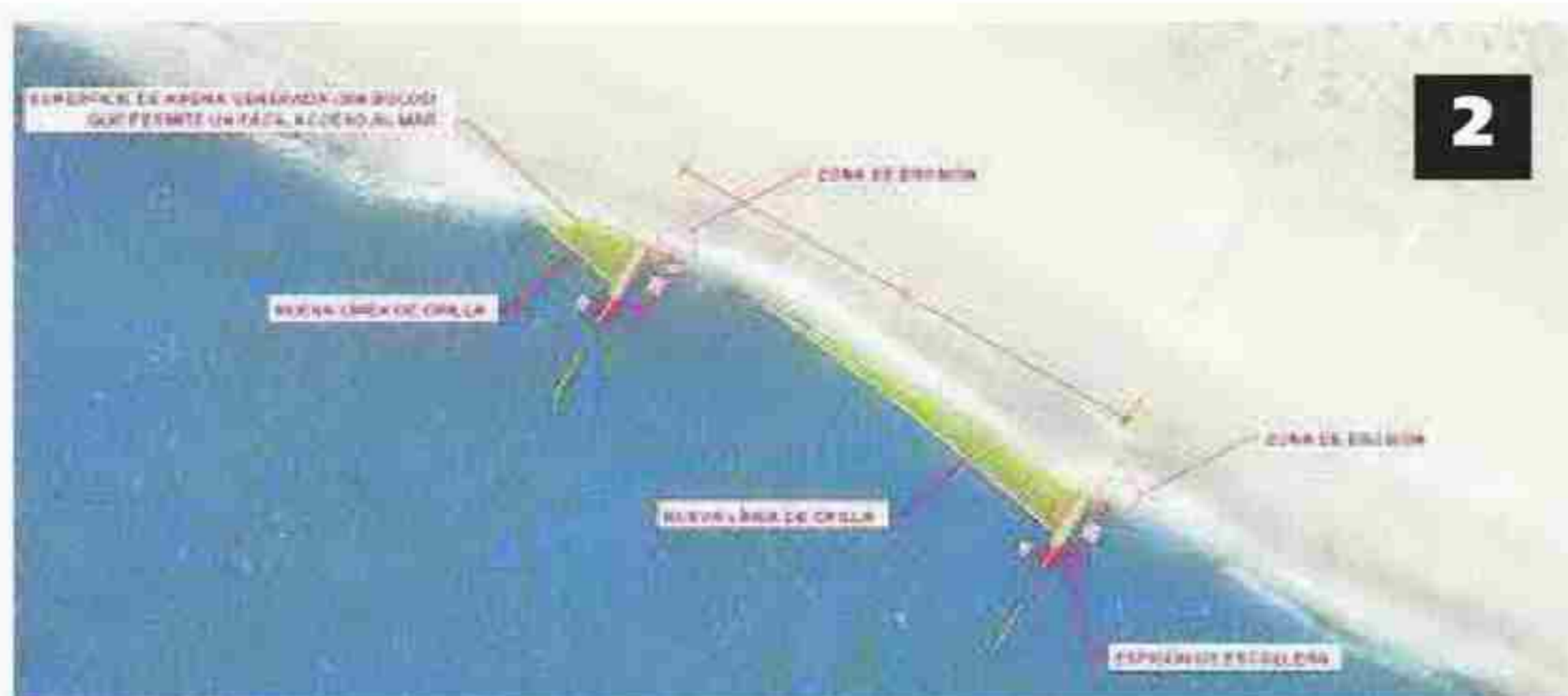
▲ Espigones de 10 m. Esta solución es la más económica tras la aportación de arena y se basa en la construcción de dos espigones.
