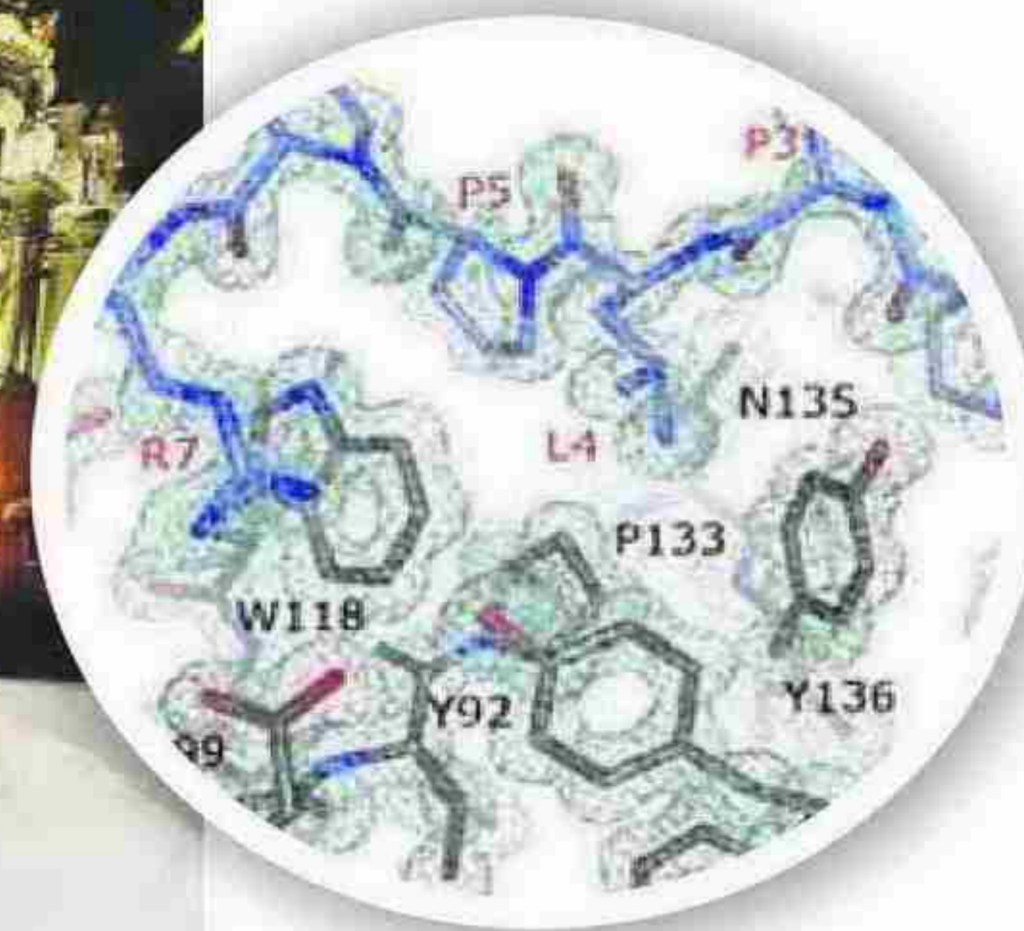
▲ Mapa de densidad electrónica.
